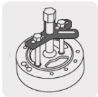
Para extraer volantes, poleas y engranes
